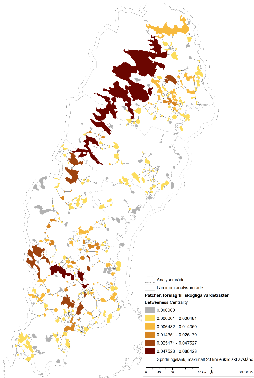
Figur 24. Betweenness Centrality av nätverksanalysen med förslag till skogliga värdestrakter.
