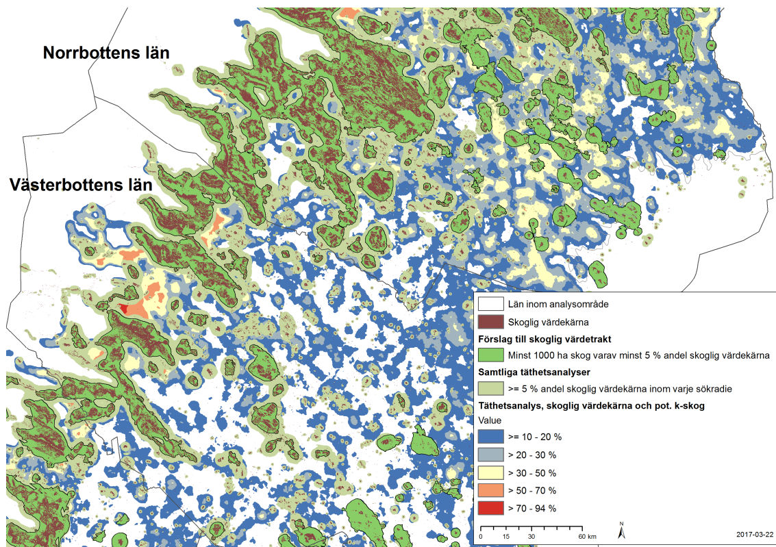
Figur 34. Karta med skogliga värdekärnor, förslag till skogliga värde-trakter, samtliga täthetsanalyser med en täthet på \geq 5\% och där en täthetsanalys av värdekärnor och kontinuitetsskogar med tätheter \geq 10\% används som visuellt stöd för att urskilja ytterligare mönster i landskapet.
