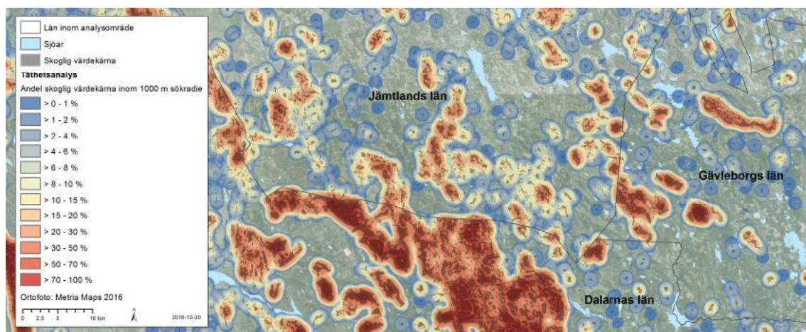
Figur 7. Täthetsanalys av skogliga värdekärnor med en sökradie på 1000 m, med kartutsnitt över bland annat Norra Mora vildmark i Dalarnas län samt Stora Sundsjöbergets och Stora Korpimäkis naturreservat i Gävleborgs län.
