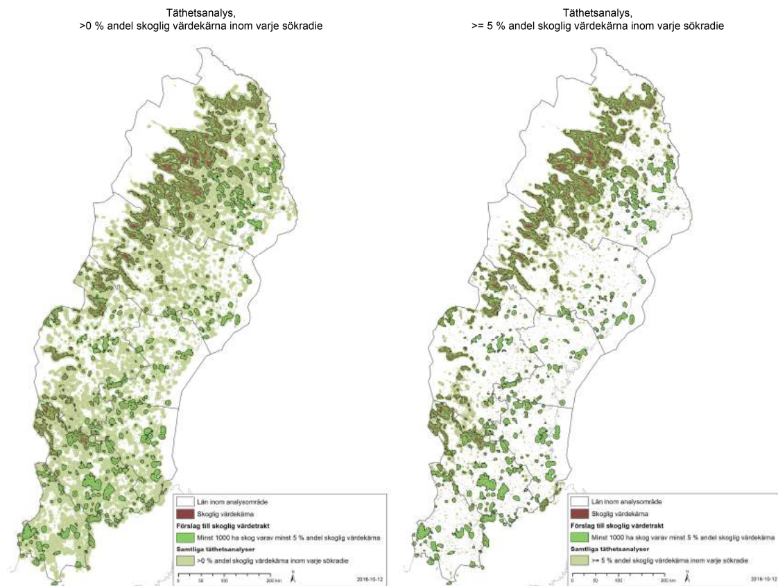
Figur 31. Synteskartor med samtliga täthetsanalyser med olika tröskelvärden. Till vänster syns alla tätheter >0\% andel skoglig värdekärna inom varje sökradie, och till höger syns tätheter \geq 5\% andel skoglig värdekärna inom varje sökradie.
