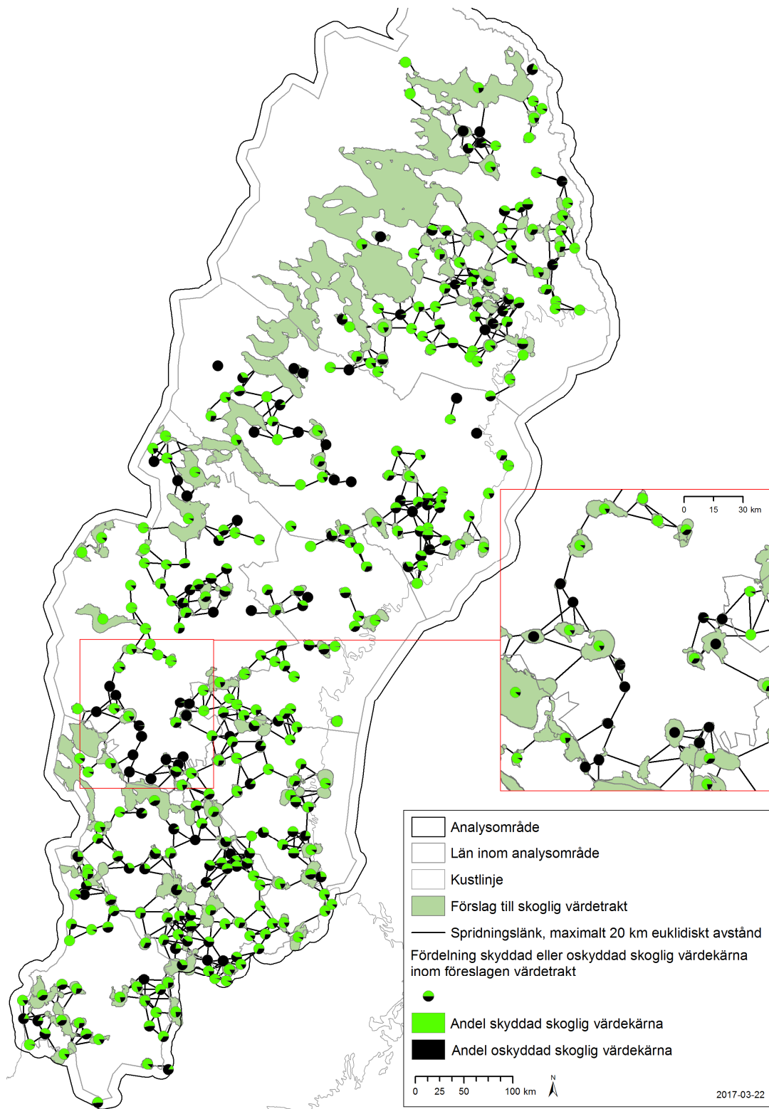
Figur 32. Synteskarta som visar förslag till skogliga värdeetrakter, spridningslänkar på ett maximalt euklidiskt avstånd på 20 km och statistik av andel skyddad eller oskyddad skoglig värdekärna inom varje trakt.
