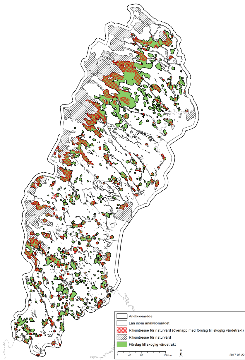
Figur 30. Jämförelse mellan förslag till skogliga värdeetrakter och överlapp med områden av riksintresse för naturvård.
