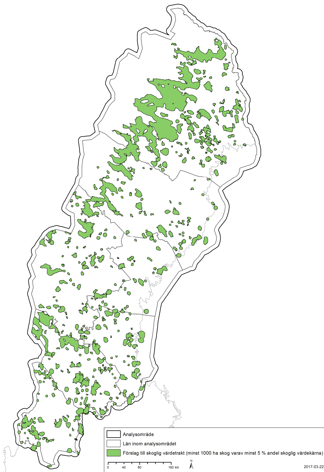
Figur 12. Förslag till skogliga värdetrakter avgränsade ur ett skogsbiologiskt och naturgeografiskt perspektiv.
