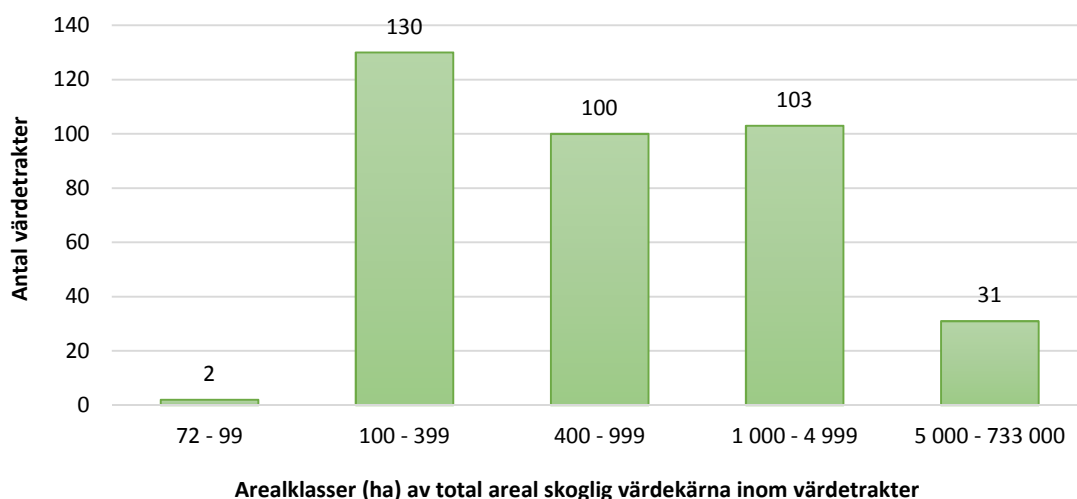
Figur 13. Diagram som visar fördelning av arealklasser (ha) av total areal skoglig värdekärna inom de olika värdeetrakterna.
