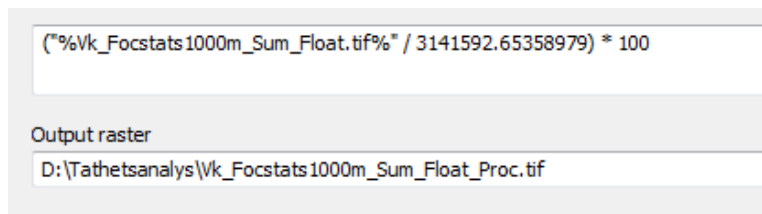
Figur 36. Skärmdump som visar inställningar i Raster Calculator för att ta fram andelar skogliga värdekärnor inom angiven sökradie (sökcirke).
