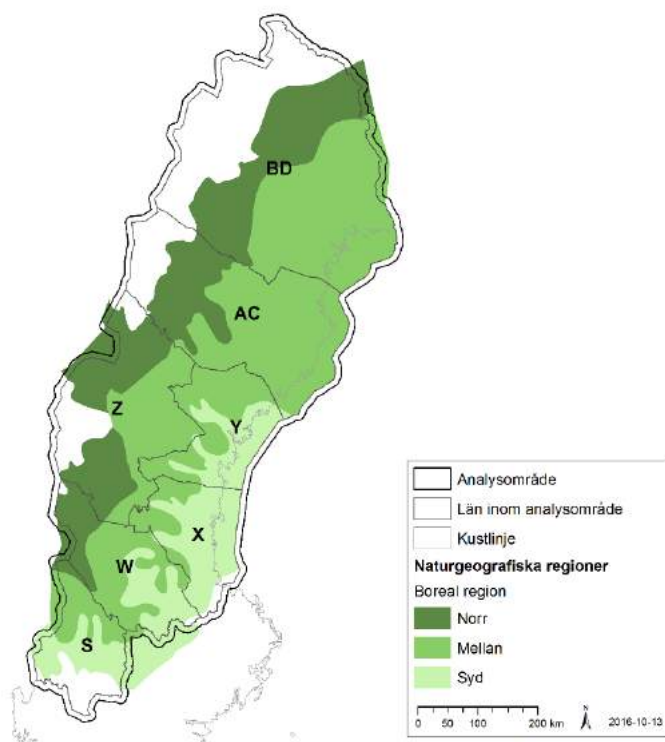
Figur 1. Översiktskarta av analysområdet och berörda län i den boreala regionen.
