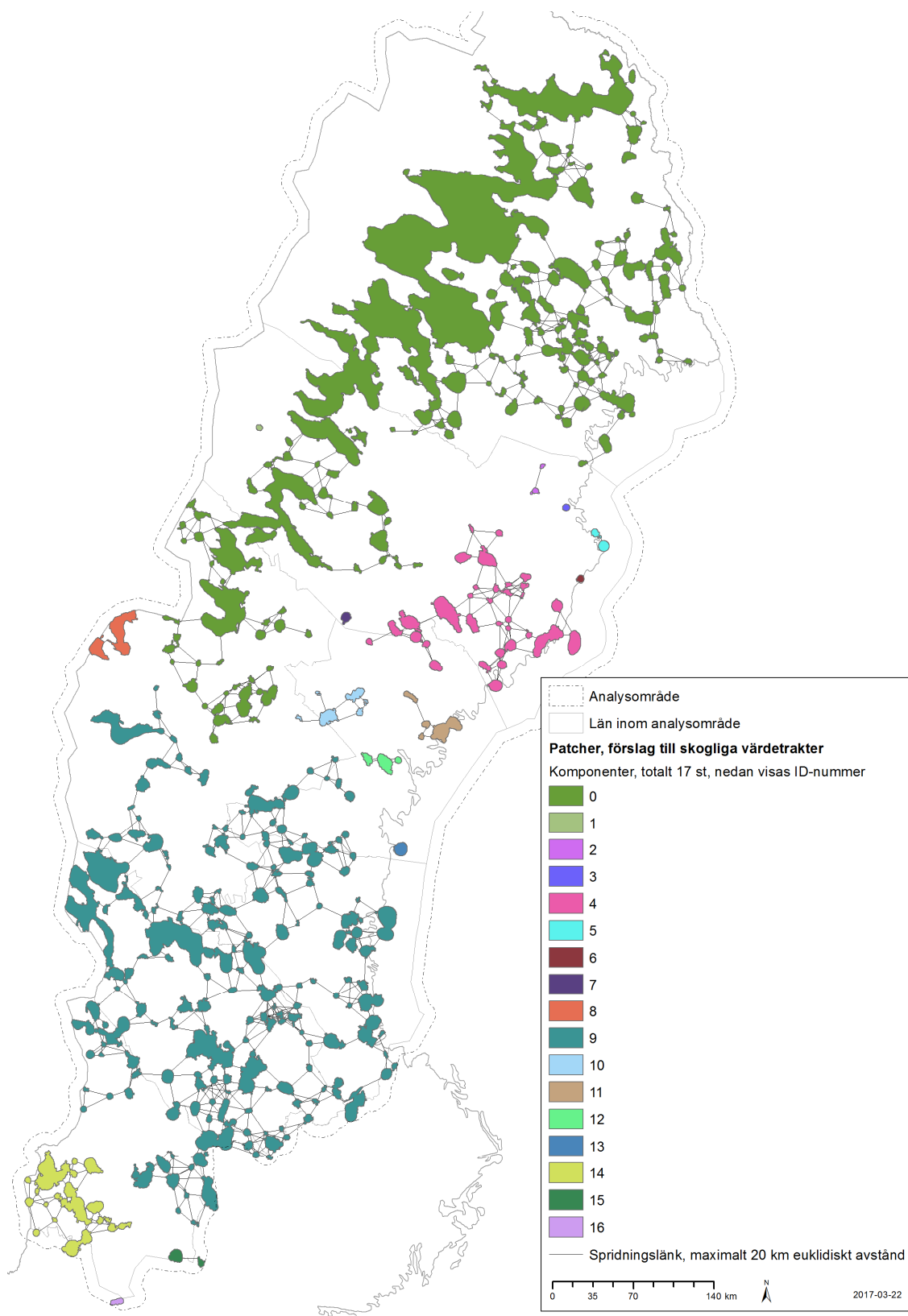
Figur 25. Komponentanalys av nätverksanalysen med förslag till skogliga värdestrakter.
