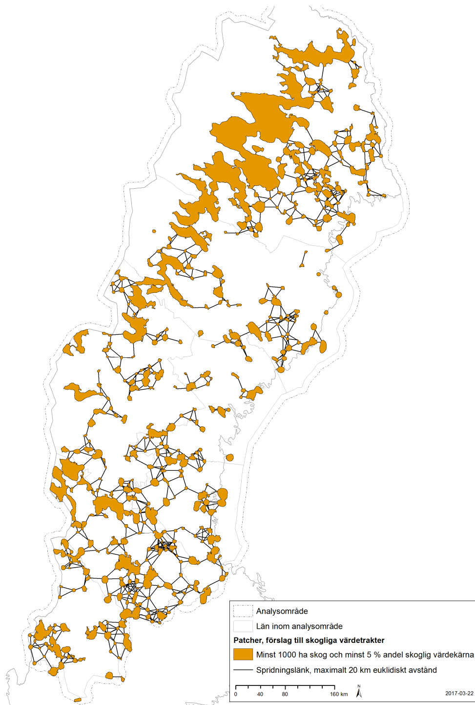
Figur 23. Nätverksanalys av förslag till skogliga värde-trakter med ett maximalt spridningsavstånd på 20 km.
