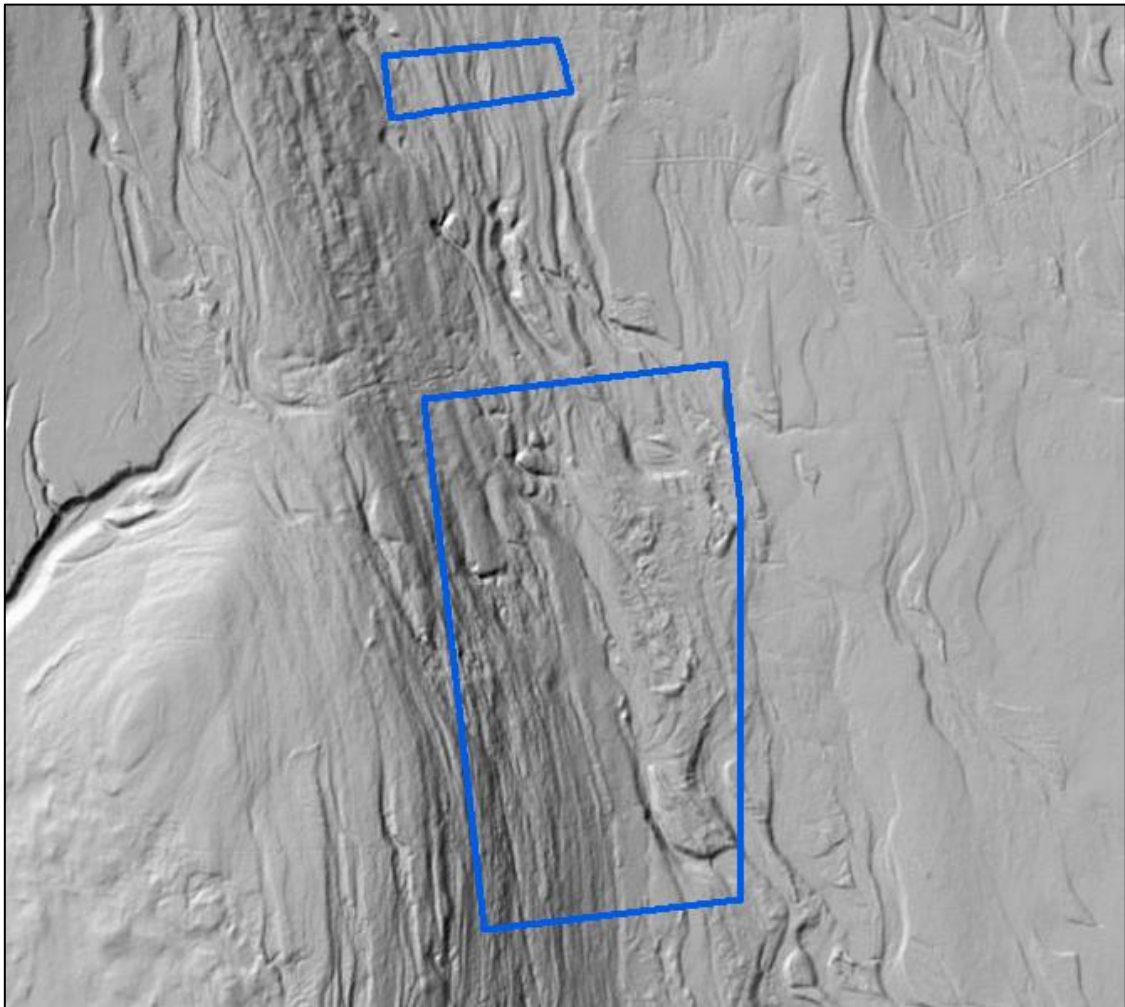
Terrängskuggningsmodell över reservatet.
