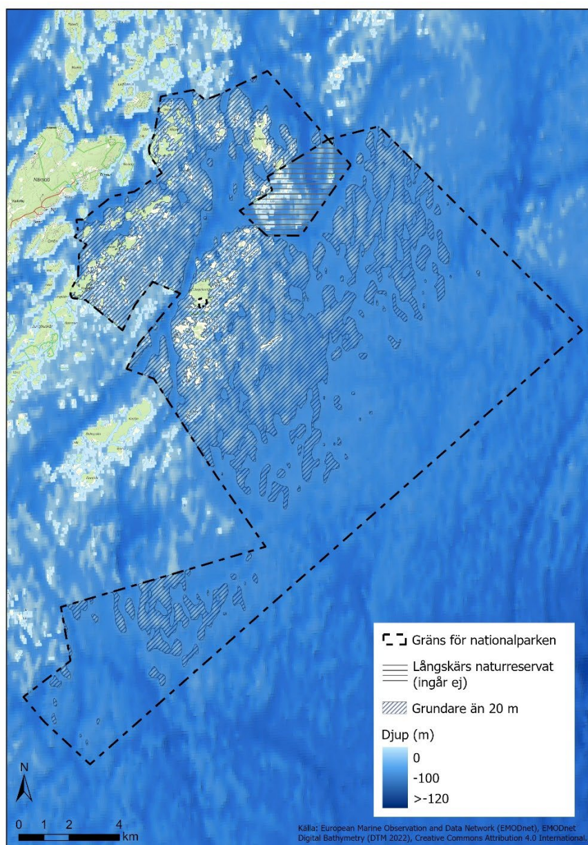
Figur 3. Översiktskarta över djupförhållanden inom och kring Nämndöskärgårdens nationalpark. Randiga områden är grundare än 20 meter. Mörkblåa/lila områden är djupast.
