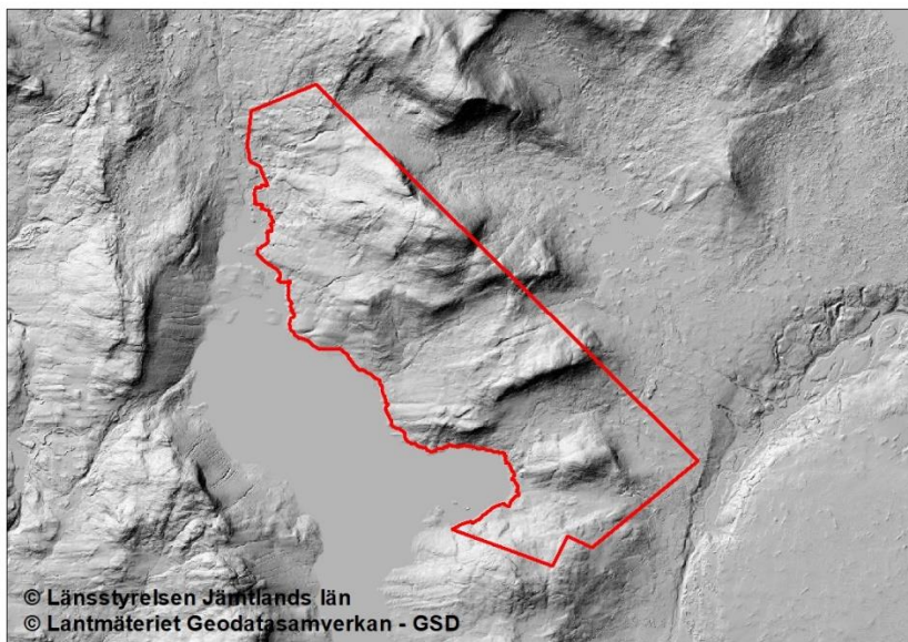
Höjdsuggningsmodell som tydliggör landskapets terrängformer.
