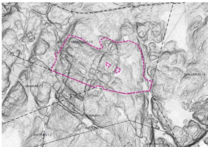
Fig. 1. Sprickdalar och branter som korsar området. (terränglutning, från nationell höjdmodell, WMS)
