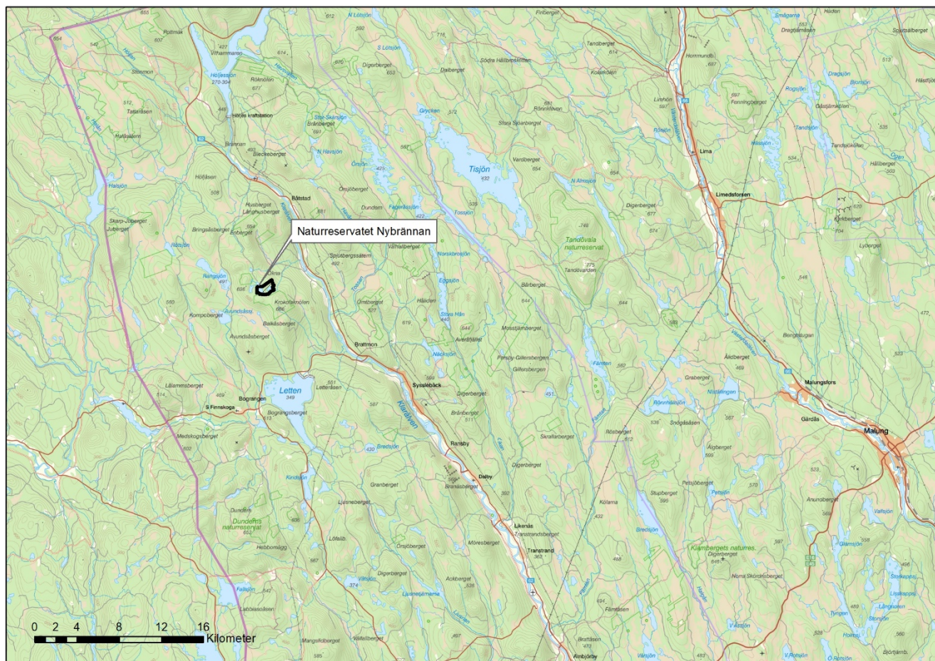
Karta 1. Översiktskarta för naturreservatet Nybrännan.
