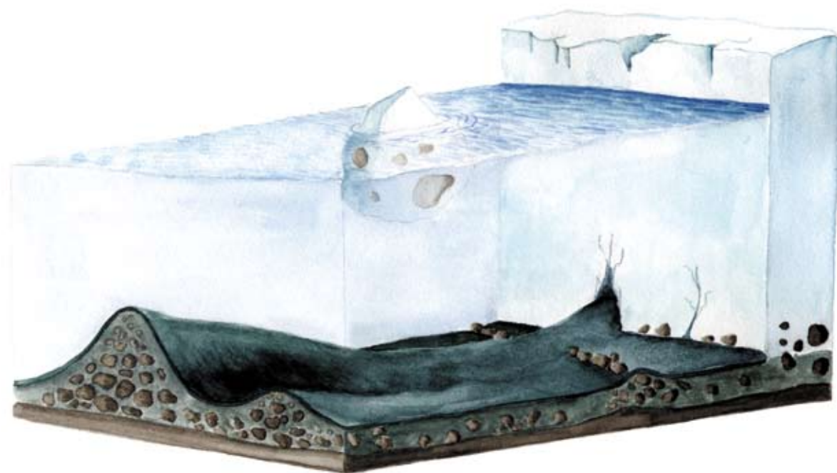
Rullstensåsar bildades när senaste inlandsisen drog sig tillbaka.
