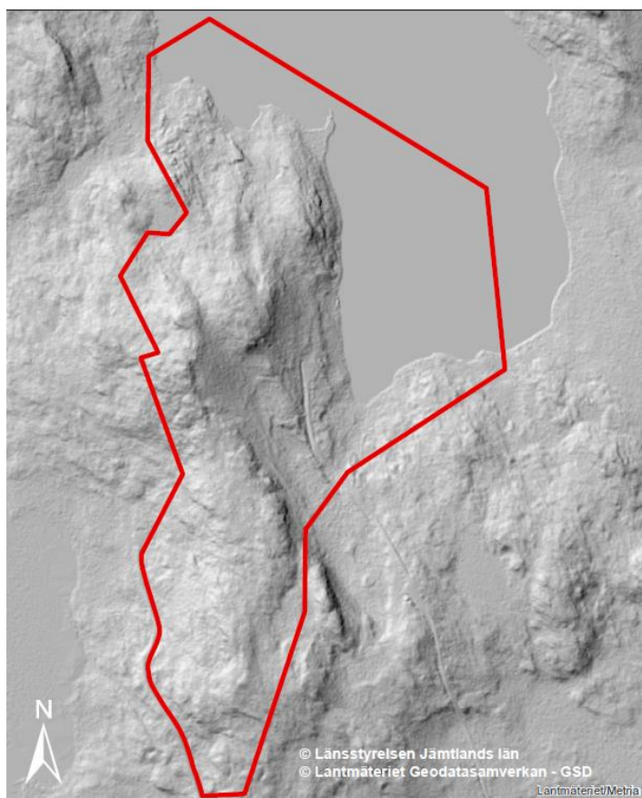
Figur 1. Höjdsuggningsmodell för tydliggörande av landskapets terrängformer inom naturreservatet Älgsjöberget.
